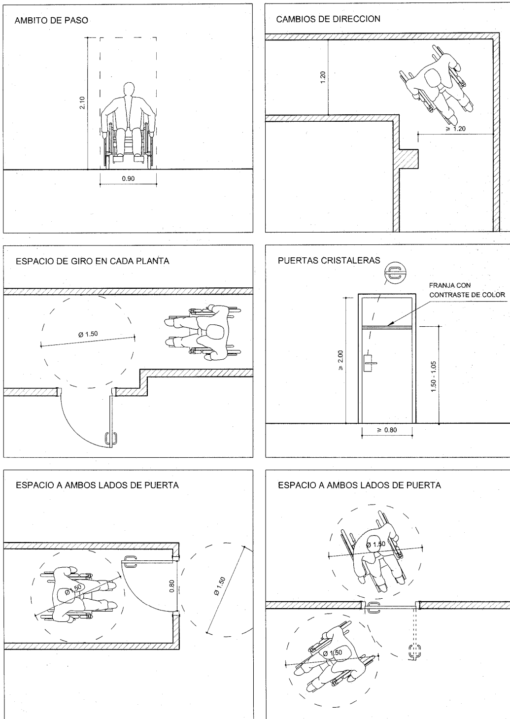
Gráficos Norma 1.E.- Itinerarios adaptados. (Interior edificios y establecimientos de uso público).
